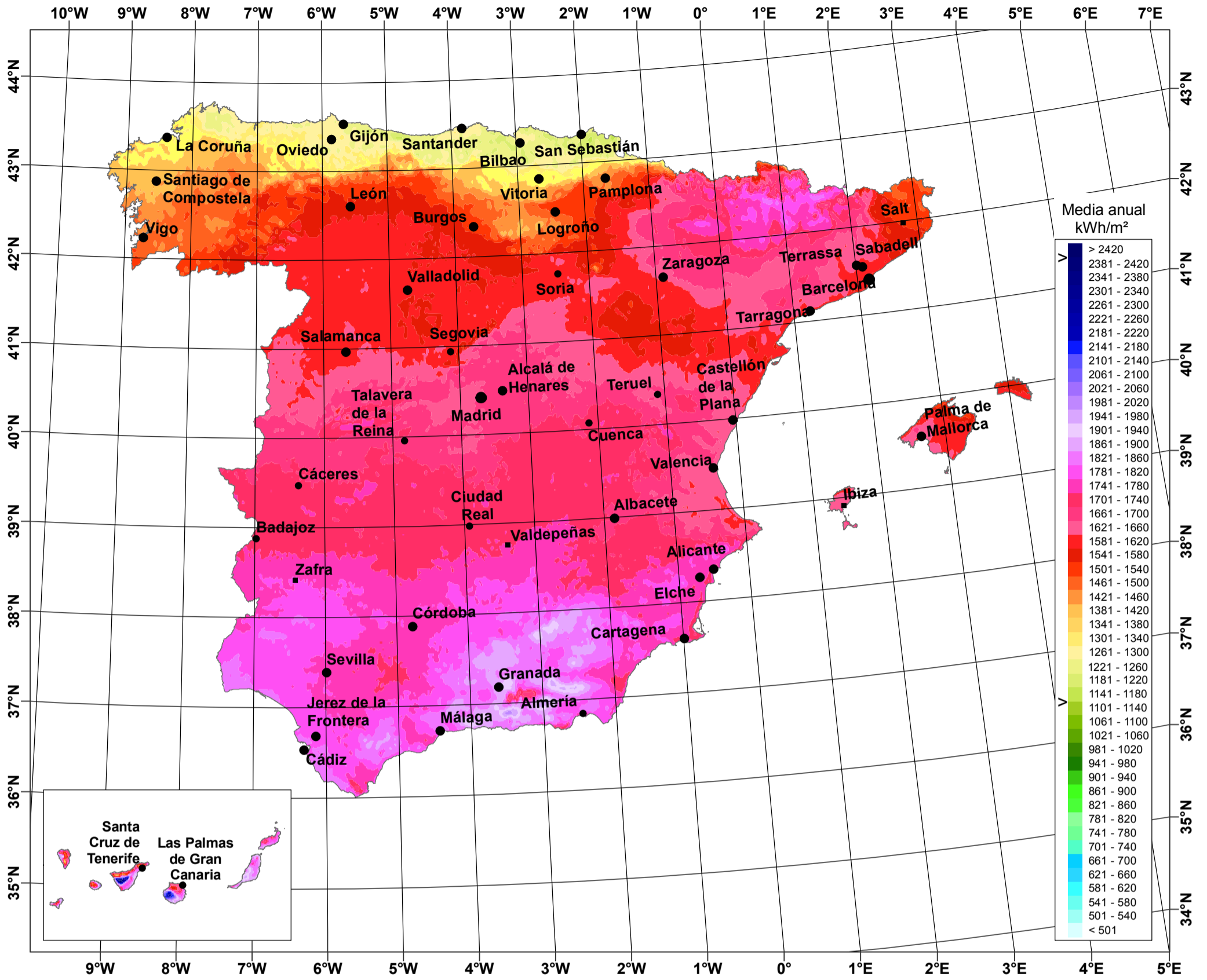
Strahlungskarte Spanien Daten: langjähriges Mittel Quelle: METEOTEST Produktion: 18.8.2008/fd
